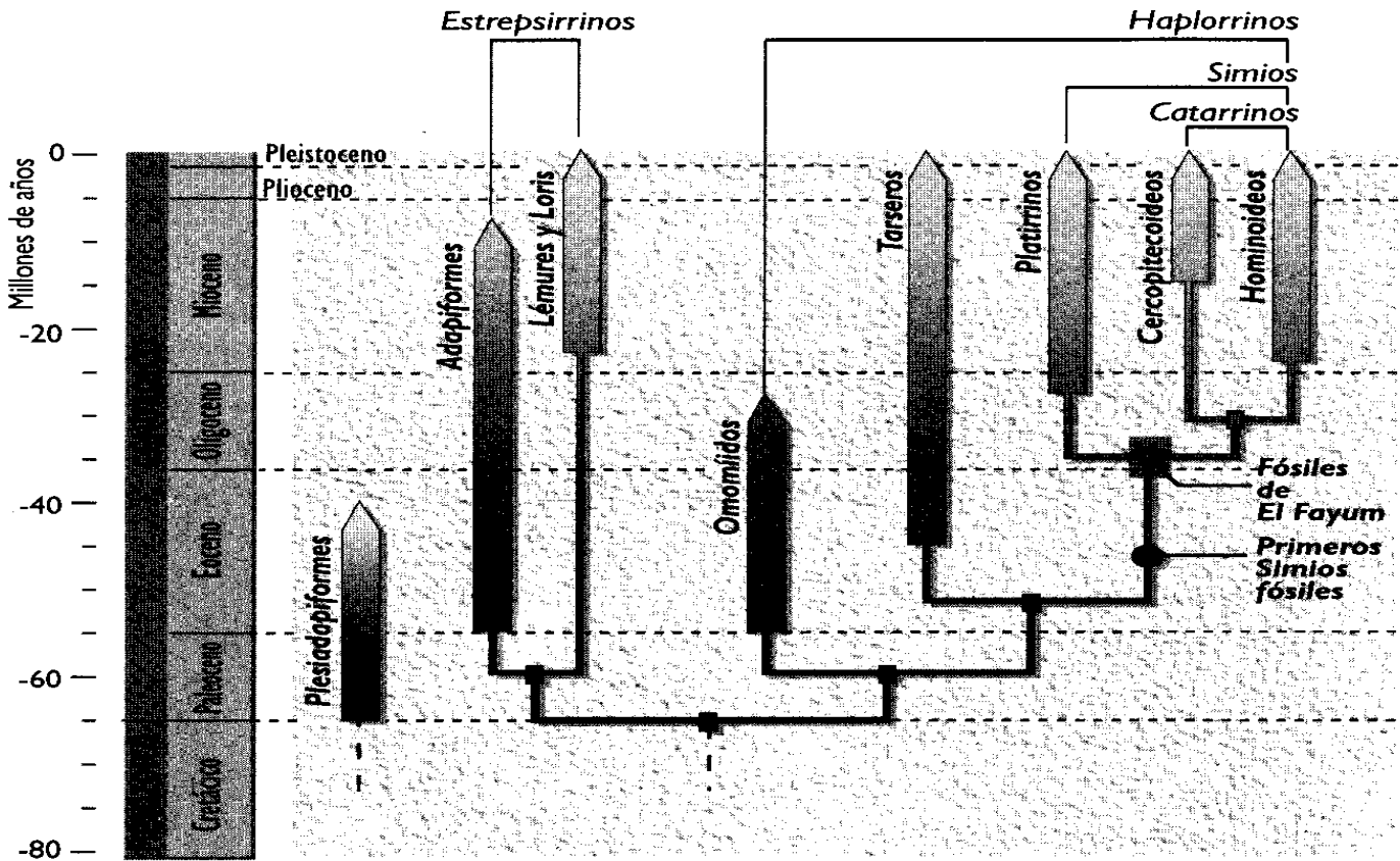
Figura 2.7. Esquema de las relaciones evolutivas de los primates.
